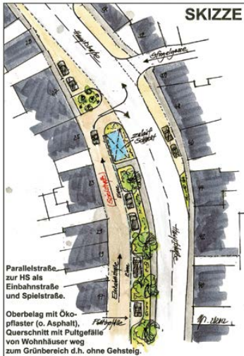
Entwurfsskizze zur Gestaltung der Lindenallee, Foto: Martin Hohm
