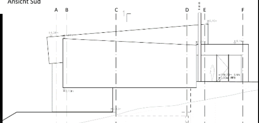
Ansicht Süd
