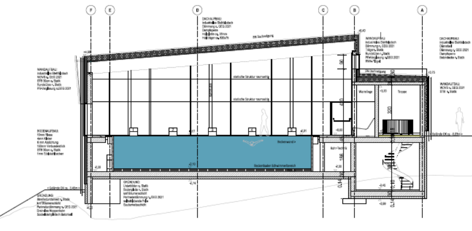
Schnitt A
